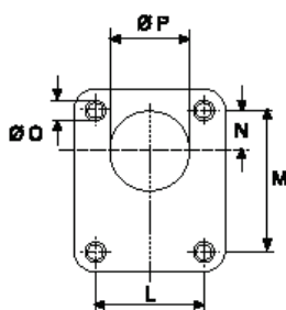
Montagem Retangular 4 furos
