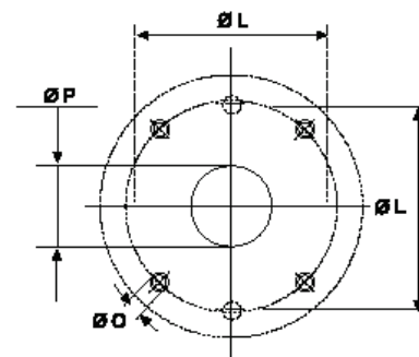
Montagem 2 furos
