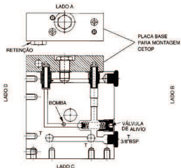
Cortes visto do lado do motor
