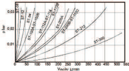
Perda de carga com óleo 36 CST/40°
