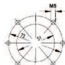
Fixação para FB-2/FBA-25
