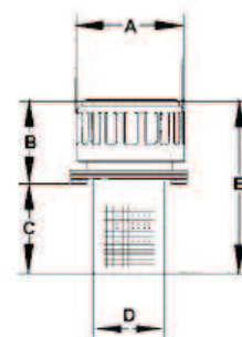
Fixação para FB-2/FBA-25
